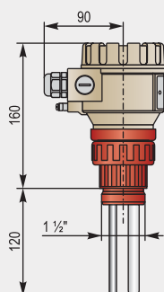
Компактный датчик + удлинитель трубы
