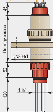
Подвесной зонд + удлинитель трубы + настраиваемый фланец
